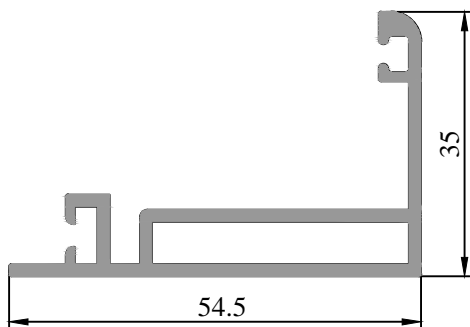
39 0302 16 0.676 kg/m
