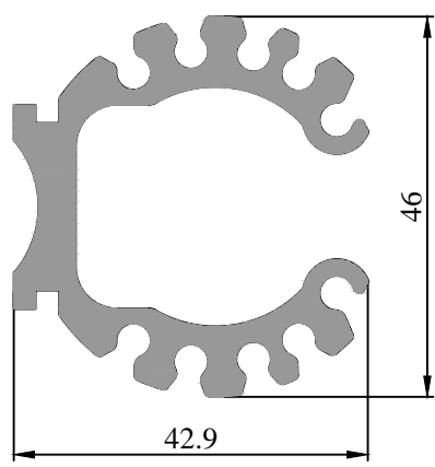
39 1607 00 1.489 kg/m
