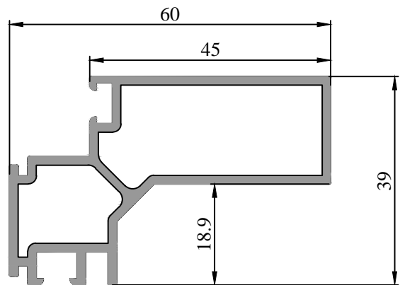
39 0301 16 0.932 kg/m
