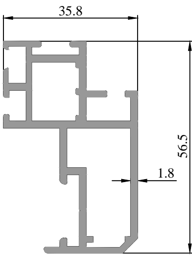
39 1301 00 1.061 kg/m.
