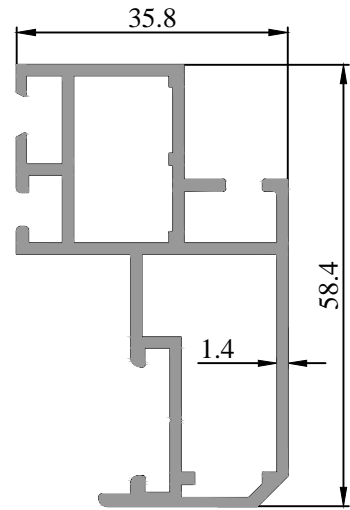
39 1303 00 0.897 kg/m.
