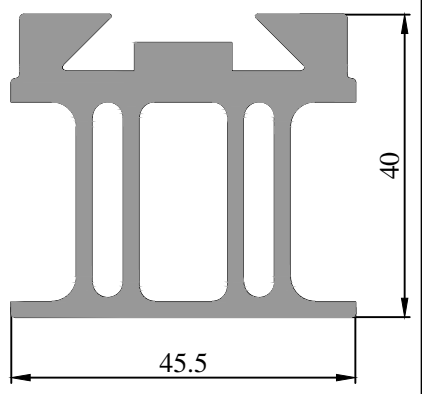
39 1608 00 1.856 kg/m
