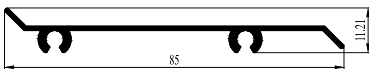
90 1991 12 0,411 kg/m.
