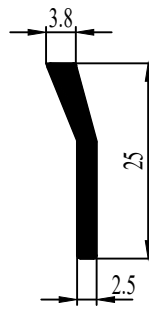
70 1590 00 0.186 kg/m.
