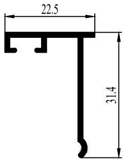
70 1589 12 0.206 kg/m.
