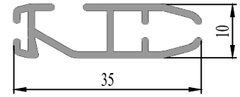
37 0747 11 0,270 kg/m.
