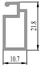
37 0736 10 0.175 kg/m.
