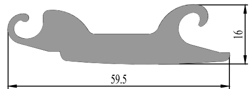
37 0741 00 1.265 kg/m.
