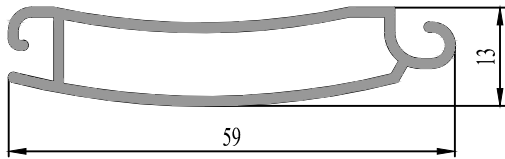
37 0716 12 0.443 kg/m.
