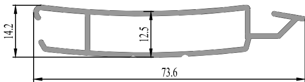
37 0726 12 0.526 kg/m.
