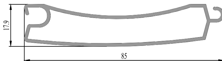
37 0725 12 0.665 kg/m.
