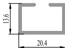
37 0721 12 0.185 kg/m.
