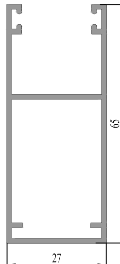
37 0739 12 0.653 kg/m.
