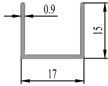
37 0753 00 0.110 kg/m.
