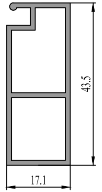
37 0761 13 0.482 kg/m.
