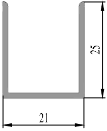
37 0702 12 0.221 kg/m.
