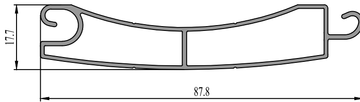
90 4940 00 0.643 kg/m.
