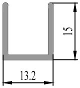
37 0720 12 0.132 kg/m.
