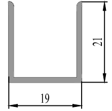
37 0703 12 0.189 kg/m.
