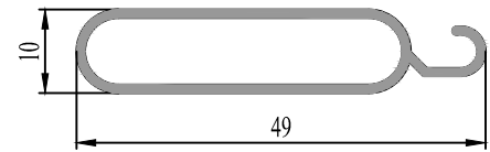
37 0705 10 0.281 kg/m.
