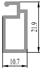
37 0736 11 0.191 kg/m.
