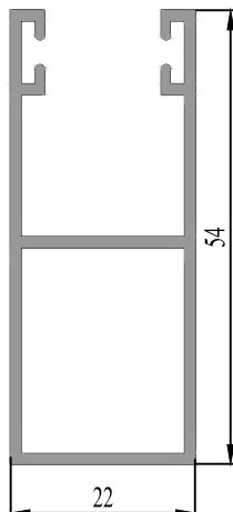
37 0717 12 0.539 kg/m.
