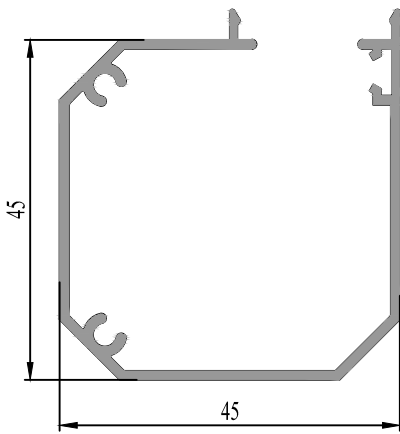
37 0745 12 0.562 kg/m.
