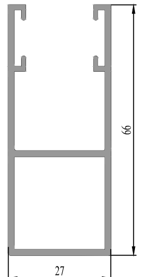
37 0708 15 0.801 kg/m.
