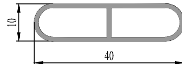
37 0729 10 0.261 kg/m.
