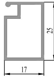
37 0737 10 0.235 kg/m.
