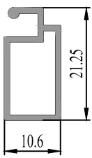
37 0760 09 0.157 kg/m.
