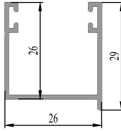
37 0701 10 0.256 kg/m.
