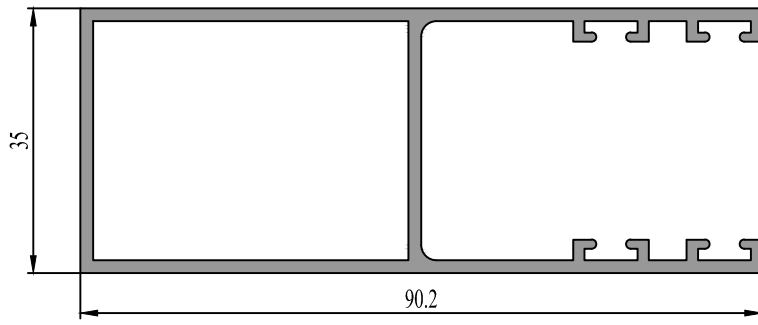
90 5022 00 1.250 kg/m.
