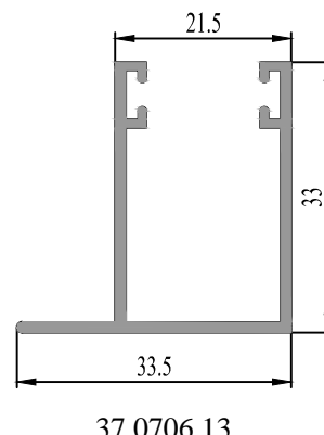
37 0706 13 0.383 kg/m.
