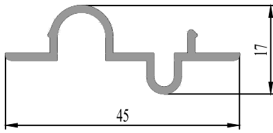
35 0623 13 : 0.261 kg/m
