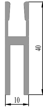
35 0605 00 : 0.434 kg/m
