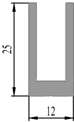
35 0603 00 : 0.357 kg/m
