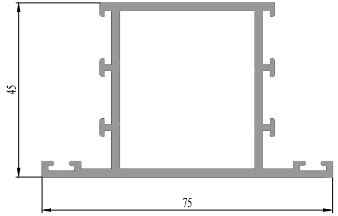
35 0627 20 : 1.211 kg/m
