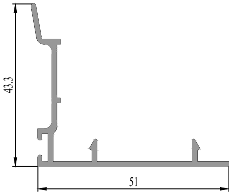
35 0609 12 : 0.385 kg/m
