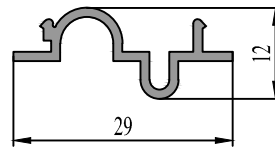
35 0618 12 : 0.171 kg/m
