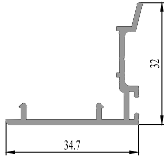
35 0616 12 : 0.279 kg/m
