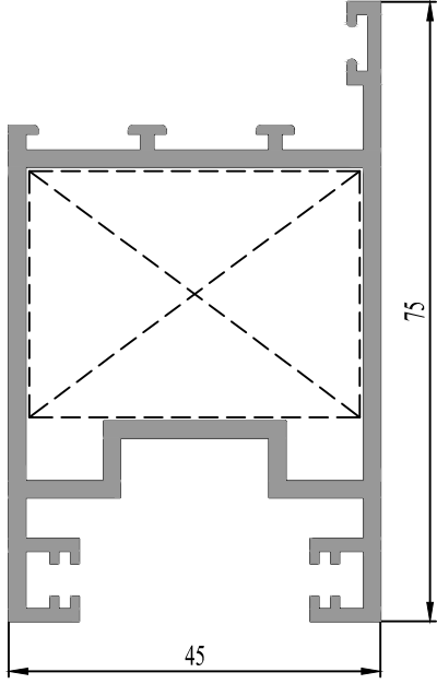
35 0601 20 : 1.451 kg/m
