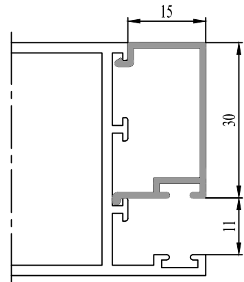
35 0610 10 : 0.204 kg/m
