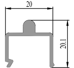
35 0608 12 : 0.222 kg/m
