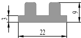
35 0606 00 : 0.339 kg/m
