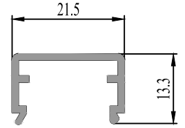
35 0626 12 : 0.170 kg/m
