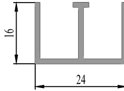
35 0604 12 : 0.232 kg/m
