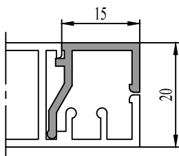
35 0628 15 : 0.174 kg/m
