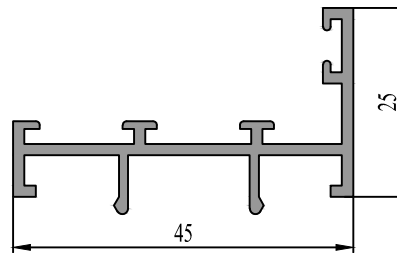
35 0619 15 : 0.452 kg/m
