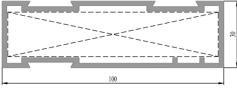
35 0602 20 : 1.520 kg/m
