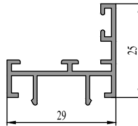
35 0613 12 : 0.319 kg/m
