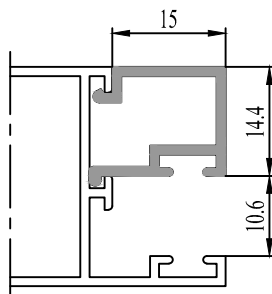
35 0615 12 : 0.190 kg/m
